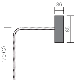
Type L Cog Bar
